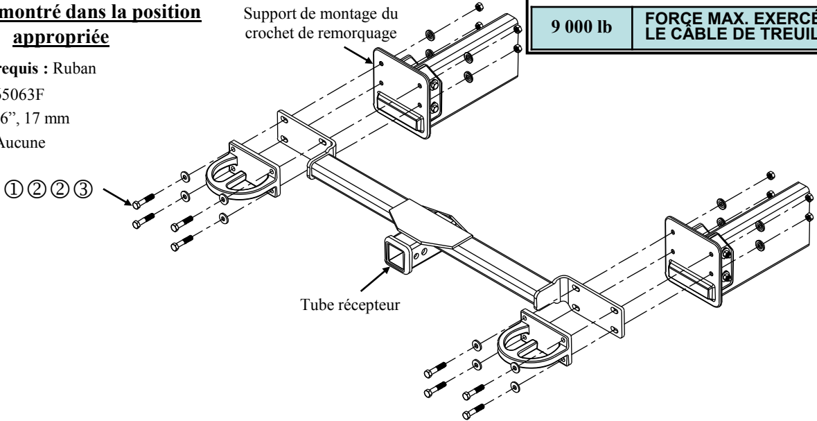
Figure 3 : Installation de l'attelage
