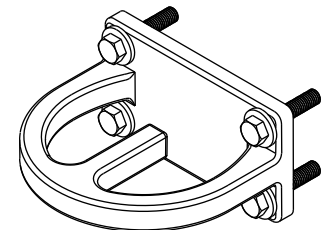
Figura 2: Ensamble de gancho de remolque OEM
