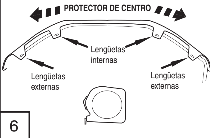
Montaje interno de la lengüeta X2
